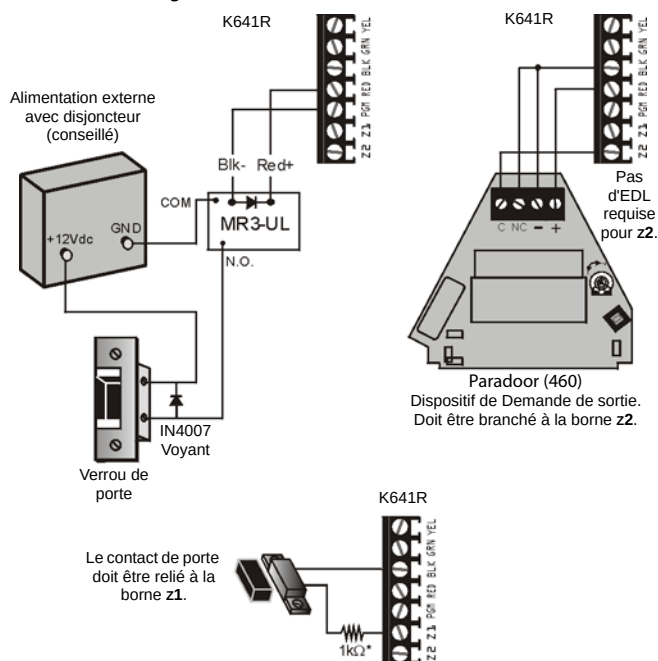
Figure 26 : : Connexion du Contrôle d'accès
