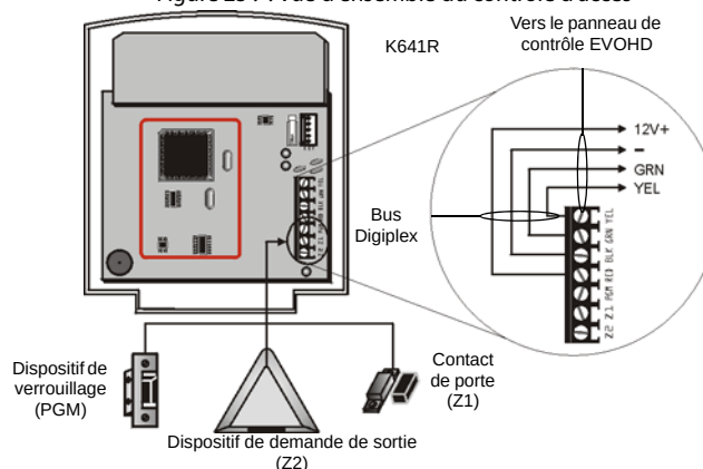
Figure 26 : : Connexion du Contrôle d'accès
