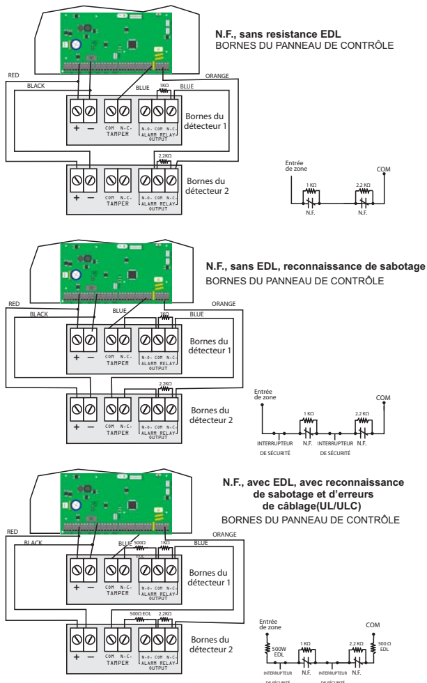
Figure 9 : Connexions de zones doublées
