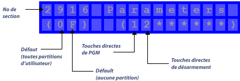
Figure 2 : Entrée de données pour section [2916] sur clavier ACL (utiliser la feuille de travail 19 à la page 38).
